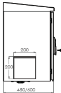
VUE DE COTE
